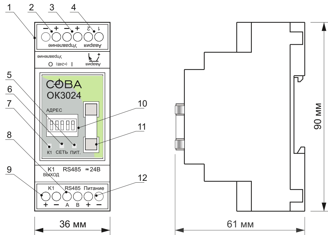
Рисунок 1. Внешний вид прибора ОК3024
