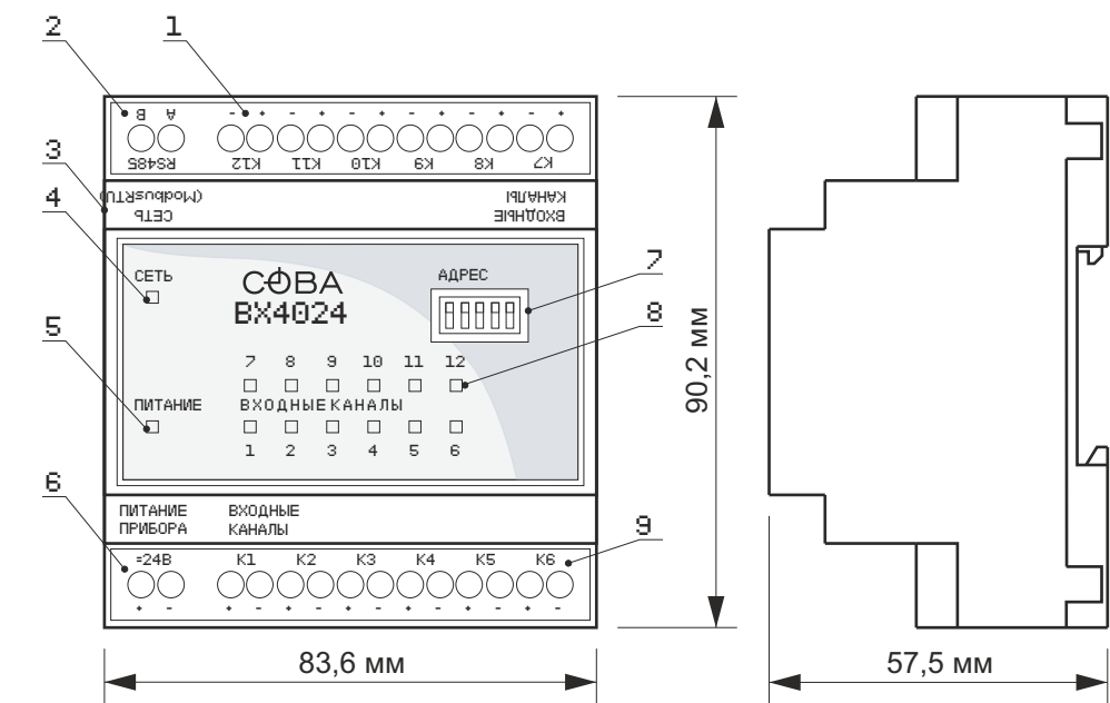
Рисунок 1. Внешний вид прибора ВХ4024
