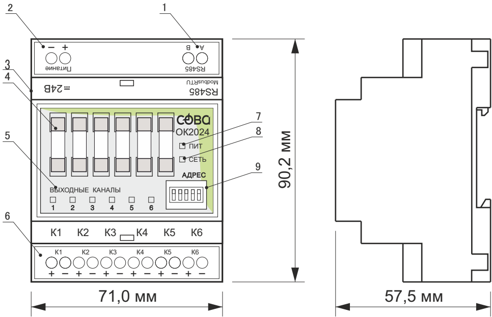
Рисунок 1. Внешний вид прибора ОК2024
