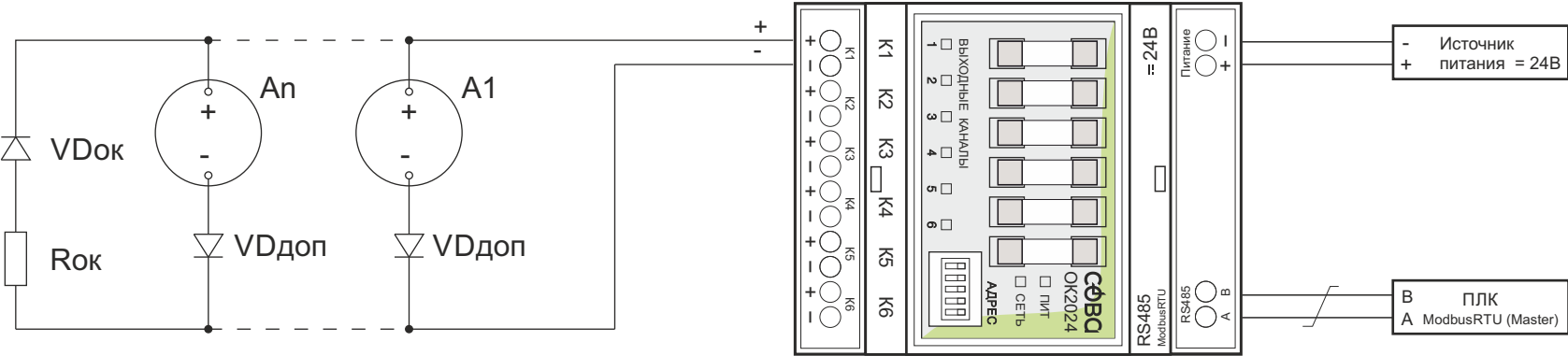
Рисунок 2. Схемы подключения «полевых» устройств. Схема организации питания, связи и передачи дискретных сигнал
